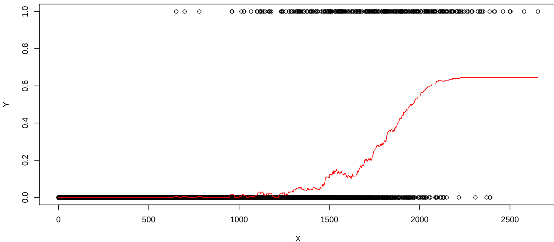
Regression KNN avec K=200
