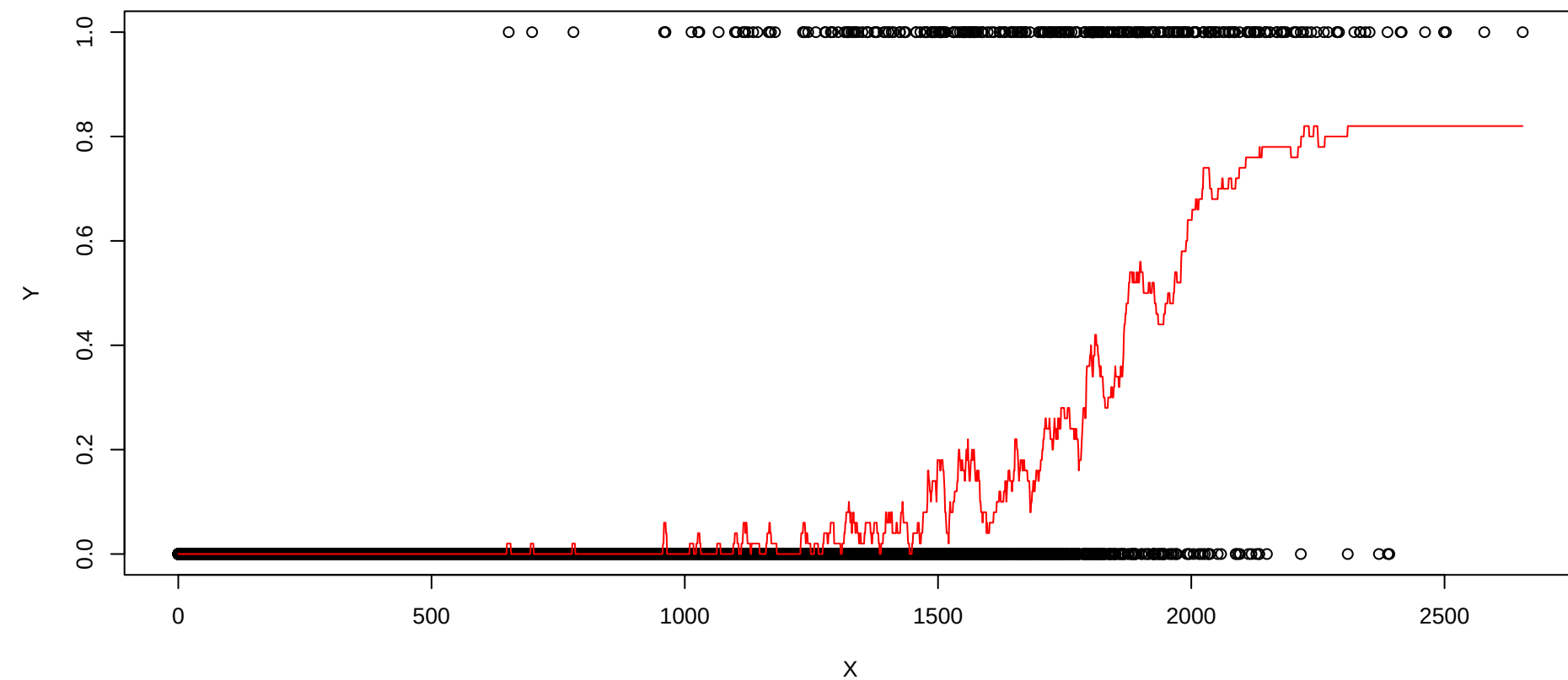
Regression KNN avec K=50
