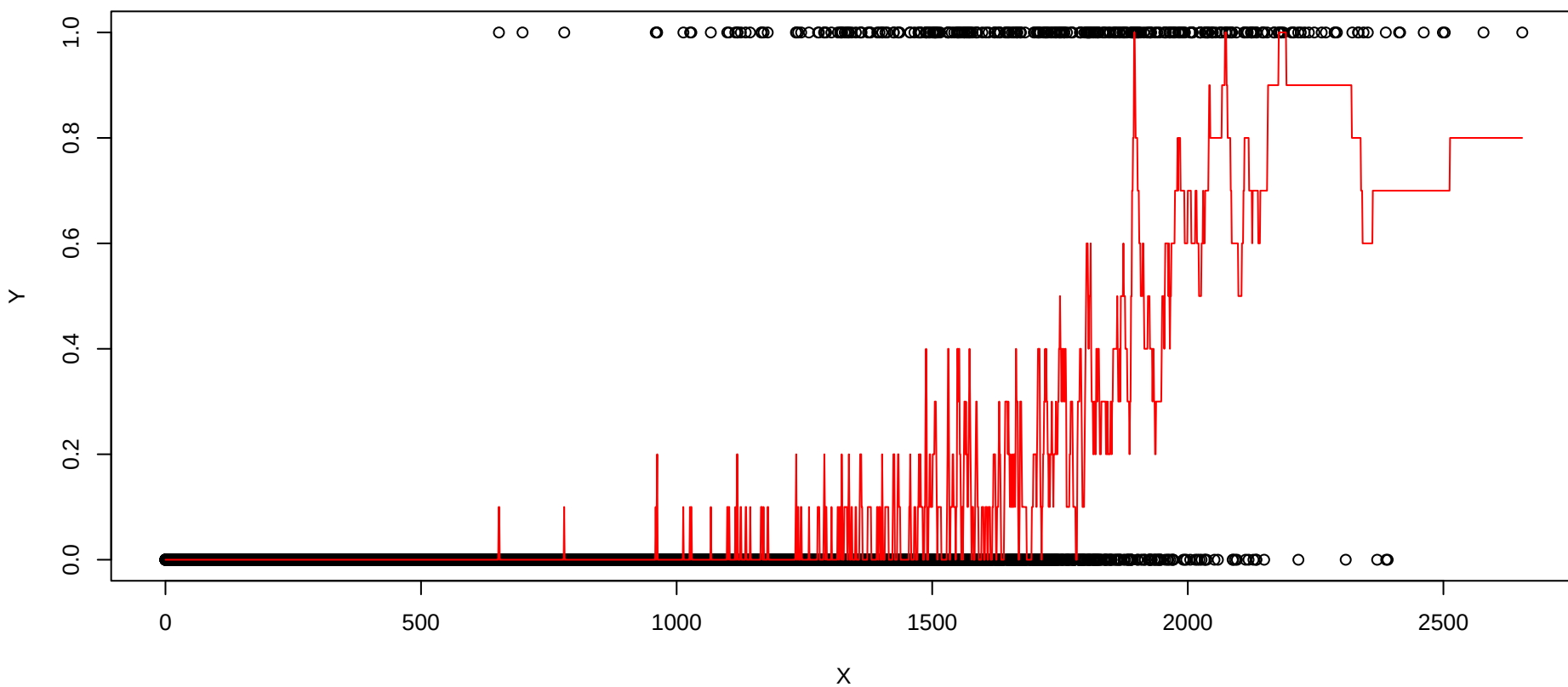
Regression KNN avec K=10
