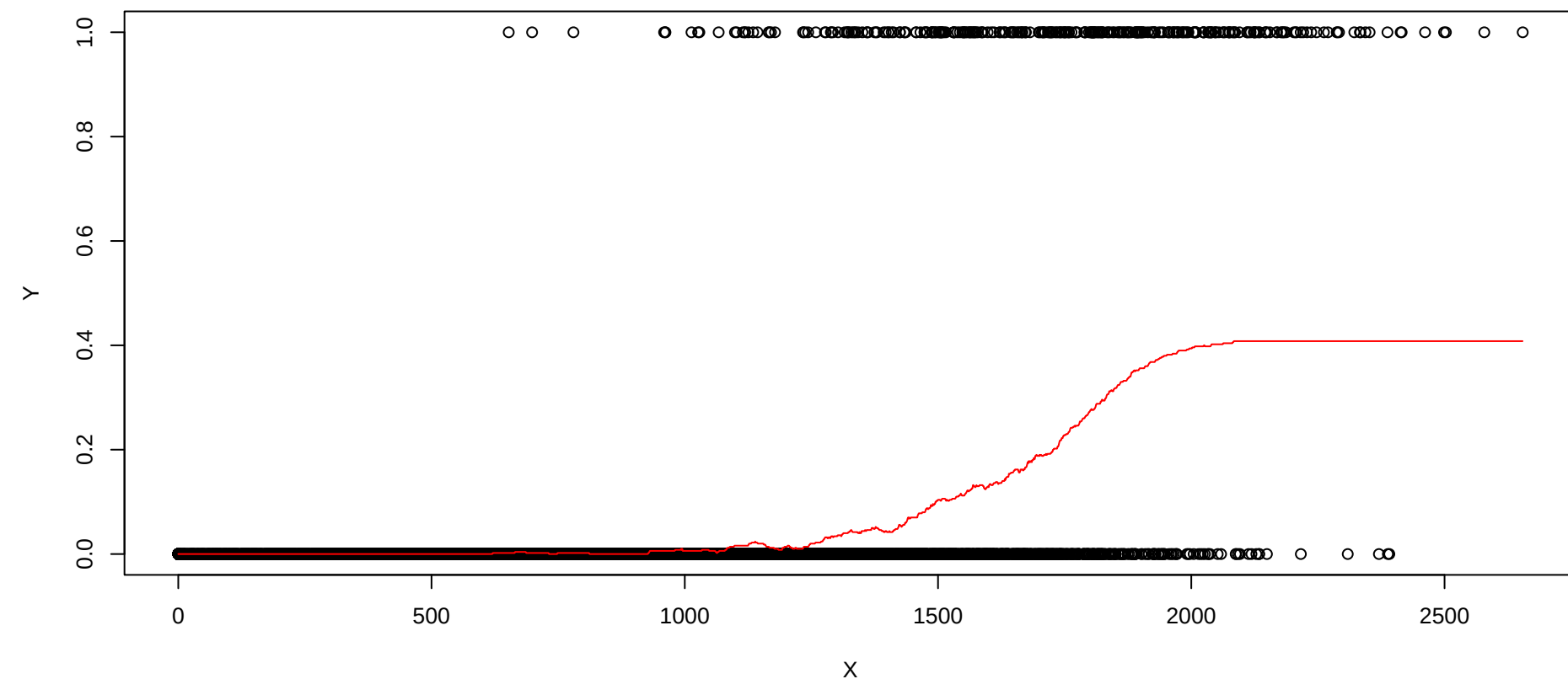
Regression KNN avec K=500
